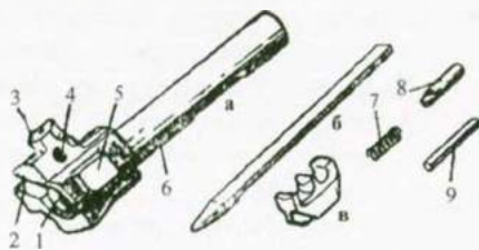
Іл. 13.4. Затвор: а — корпус затвора; б — ударник; в — викидач
