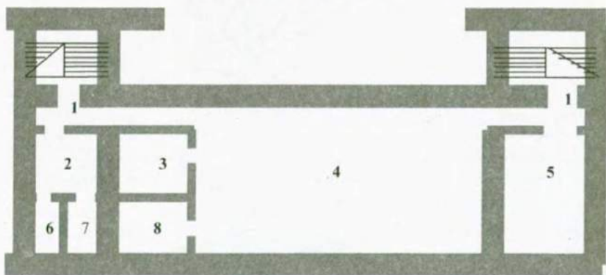
Іл. 35.4. Схема протирадіаційного укриття (варіант)
