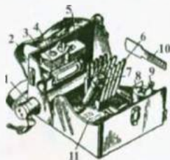
Іл. 34.10. Військовий прилад хімічної розвідки (ВІХР): 1 — ручний насос; 2 — плечовий ремінь з тасьмою; 3 — насадка до насоса; 4 — захисні ковпачки для насадки; 5 — протидимні фільтри; 6 — патрон ґрілки; 7 — електричний ліхтар; 8 — корпус ґрілки; 9 — штир; 10 — лопатка; 11 — індикаторні трубки в касетах
