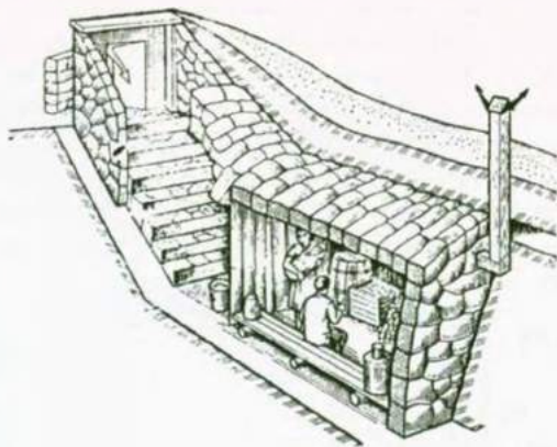
Іл. 35.2. Погріб, пристосований під ПРУ
