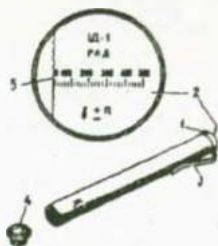
Іл. 34.8. Індивідуальний дозиметр ІД-1: 1 — окуляр; 2 — шкала; 3 — тримач; 4 — заслінка; 5 — платинова нитка
