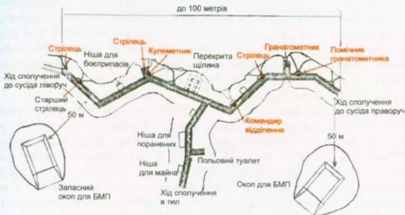
Іл. 7.3 Фортифікаційне обладнання позиції механізованого відділення на БМП
