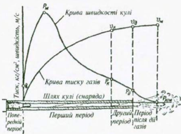
Іл. 11.1. Періоди пострілу
