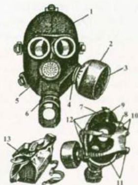
Іл. 36.7. Протигаз ЦП-7: 1 — лицьова частина;
