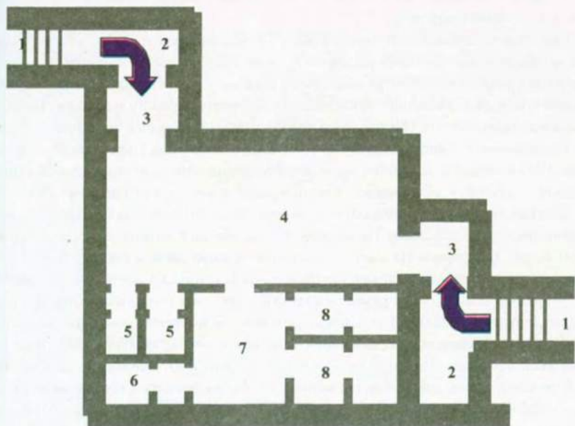
Іл. 35.5. План-схема окремо розташованого сховища:
