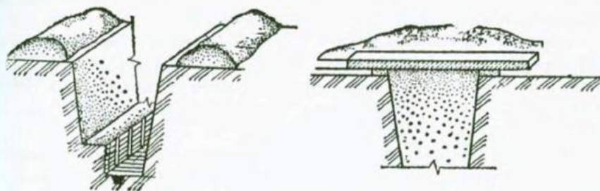
Іл. 35.1. Відкрита та перекрита щілини
